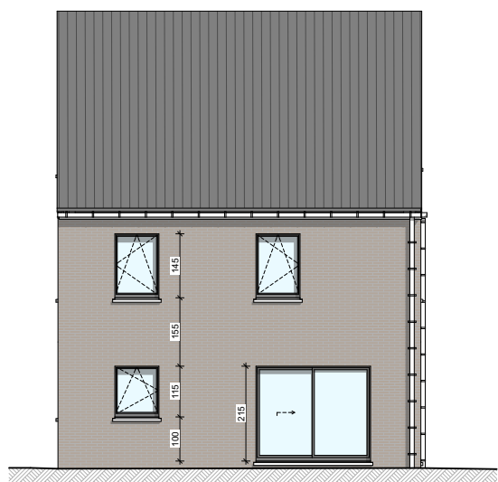
Façade arrière
