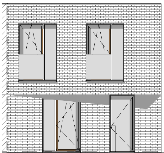
Vorgevel
