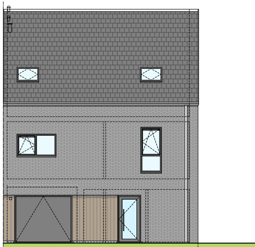
Façade avant
