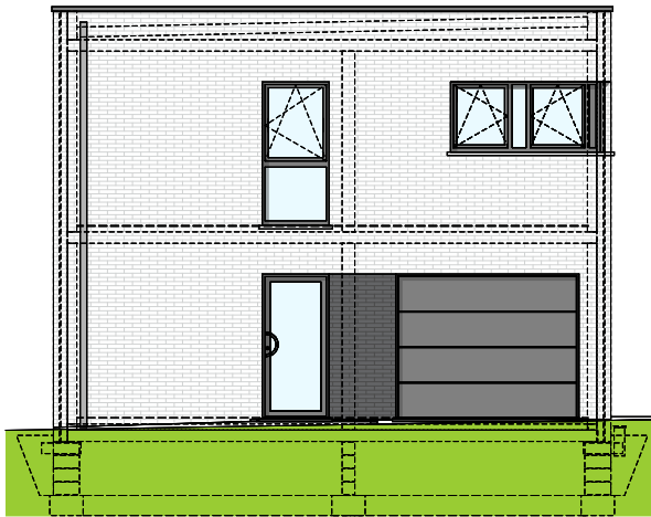
Façade avant
