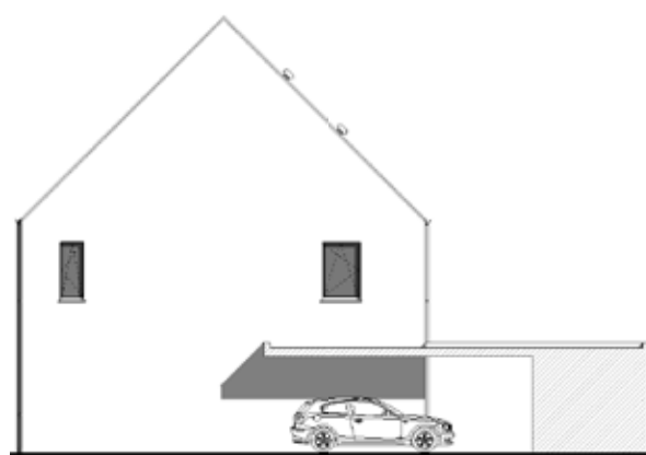
Zijgevel rechts
