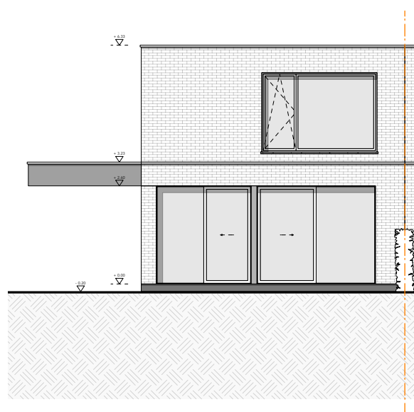
Achtergevel
