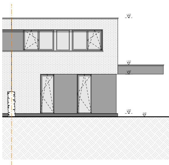
Voorgevel
