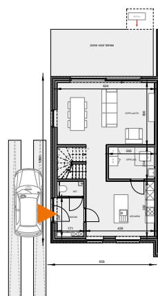
Plan gelijkvloers incl. tuin en staanplaats
