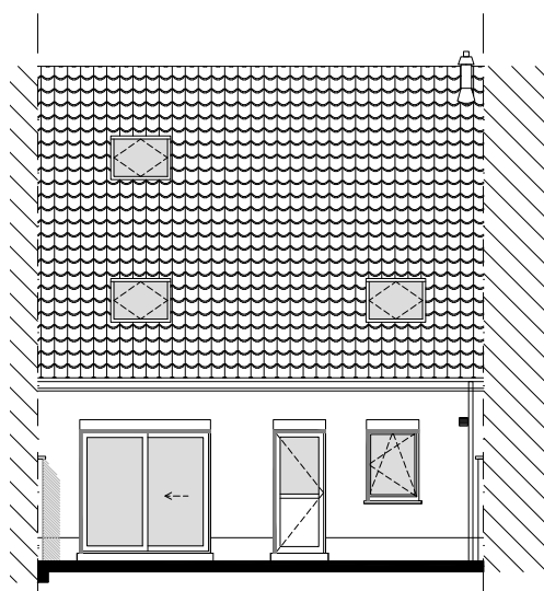
Achtergevel
