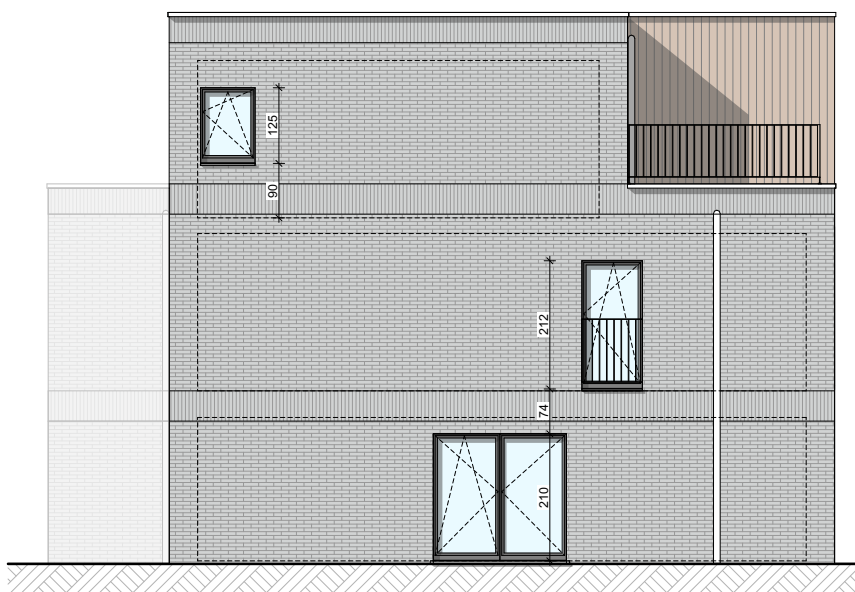
Façade latérale gauche
