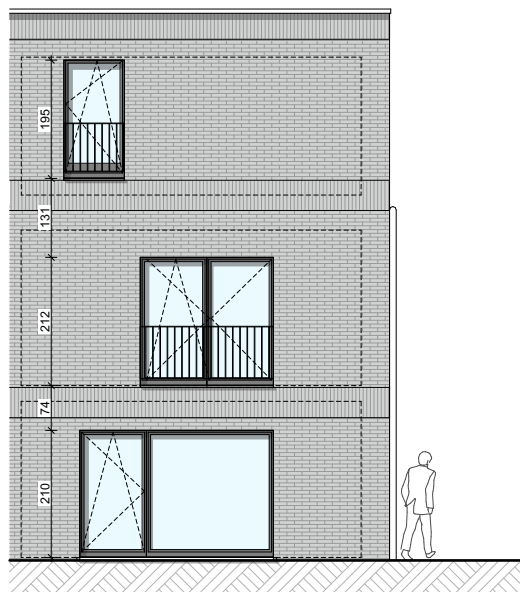
Façade arrière
