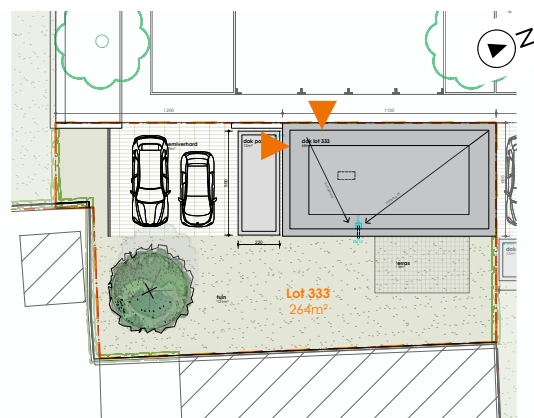
Plan gelijkvloers incl. tuin
