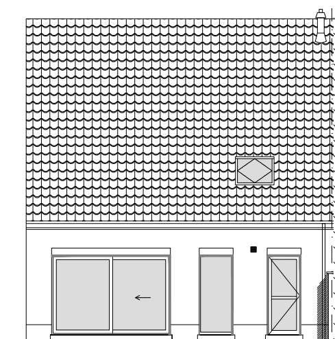
Achtergevel
