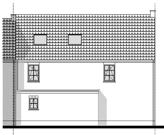
Zijgevel links
