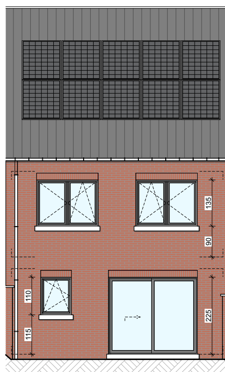
Façade arrière
