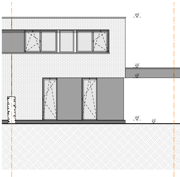
Voorgevel
