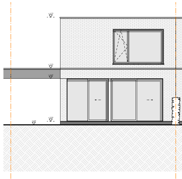
Achtergevel
