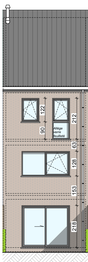
Façade arrière
