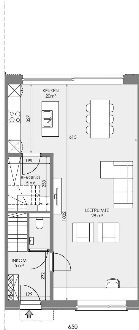
GELIJKVLOERS
