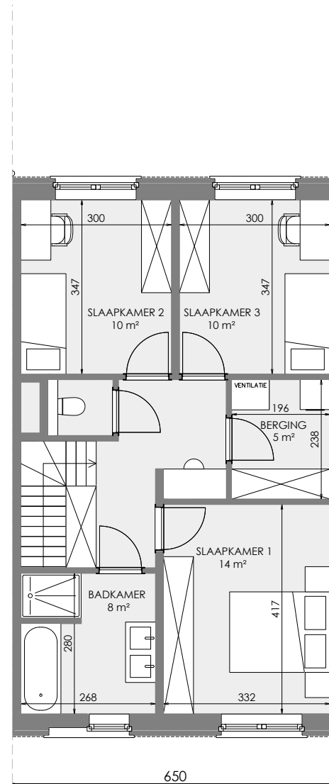
VERDIEPING 1
