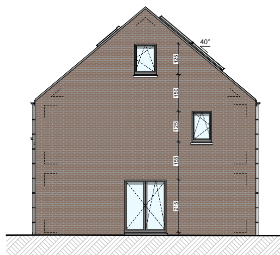
Façade latérale gauche
