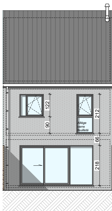
Façade arrière
