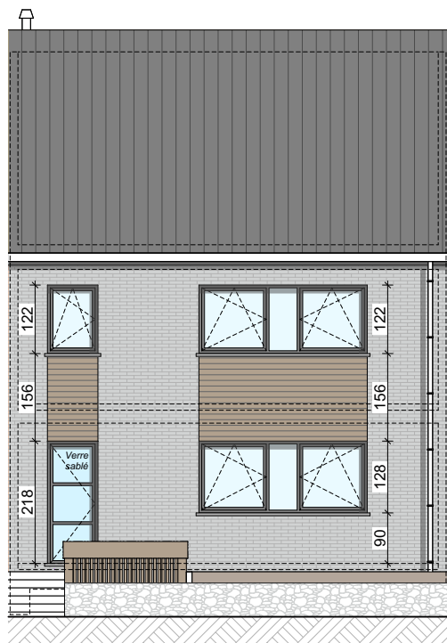
Façade avant
