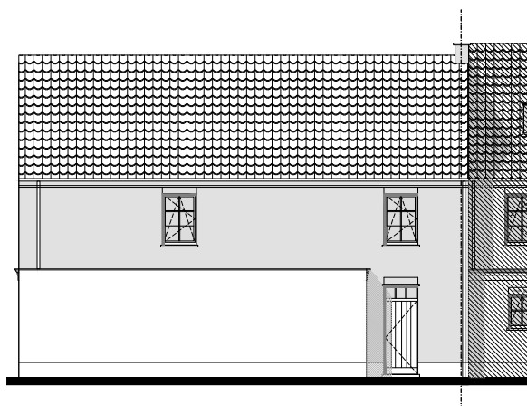
Zijgevel links
