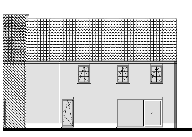
Zijgevel rechts
