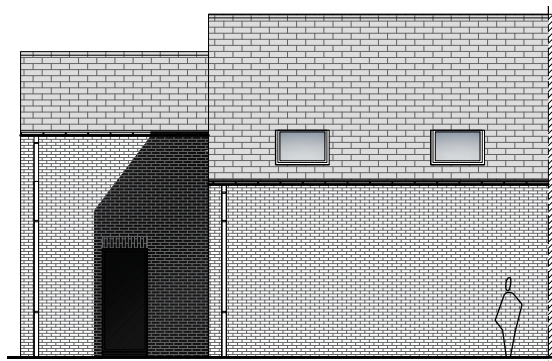
Zijgevel rechts
