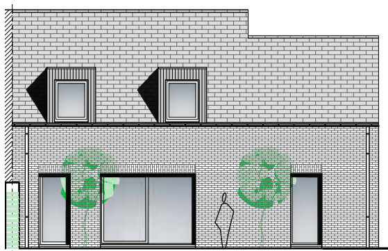
Zijgevel links
