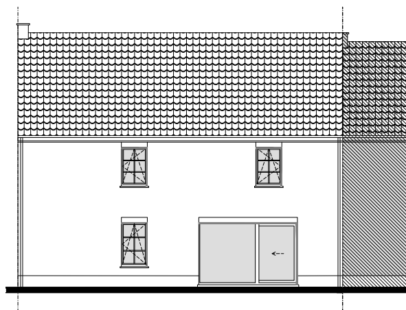
Zijgevel rechts
