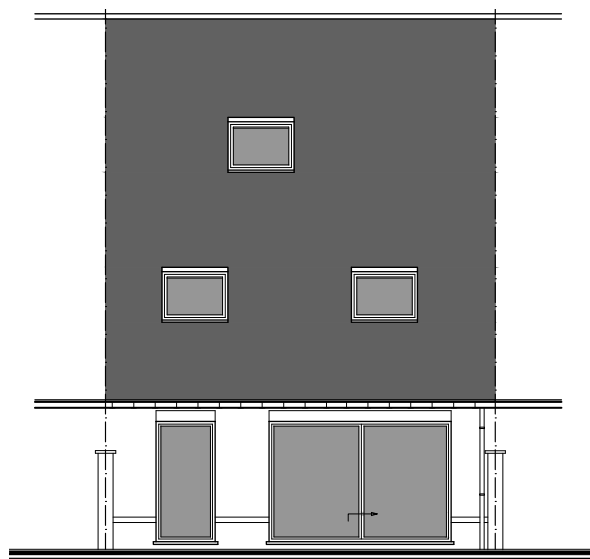
Achtergevel
