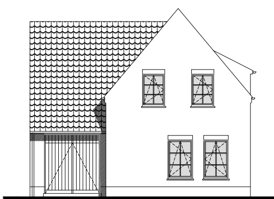
Vorgevel
