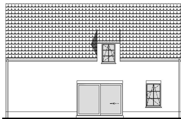
Zijgevel rechts
