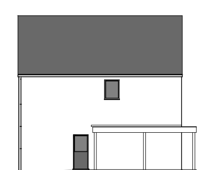
Zijgevel rechts
