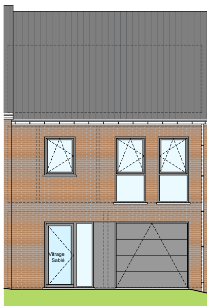
Façade avant
