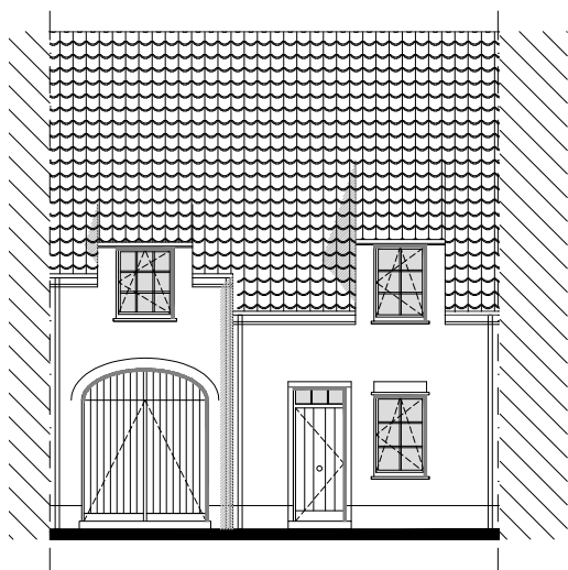
Voorgevel
