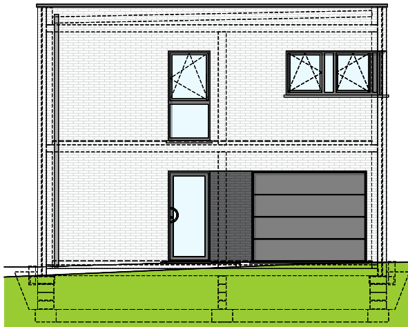
Façade avant
