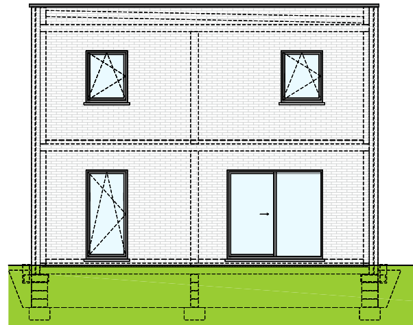
Façade arrière
