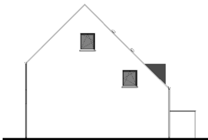
Zijgevel rechts
