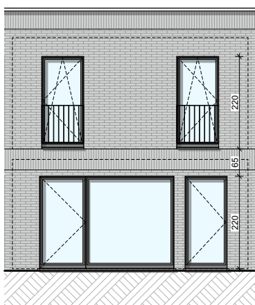
Façade arrière
