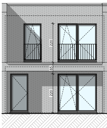
Façade avant
