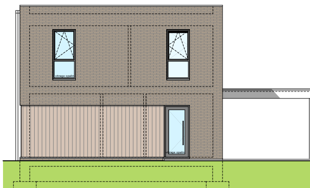
Façade avant
