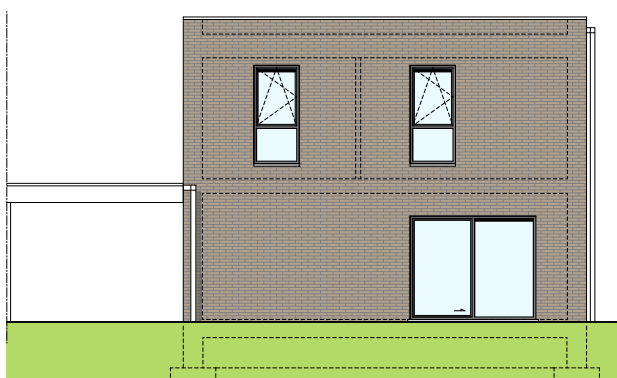
Façade arrière
