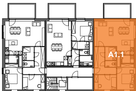
Plan général
