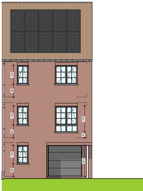
Façade avant
