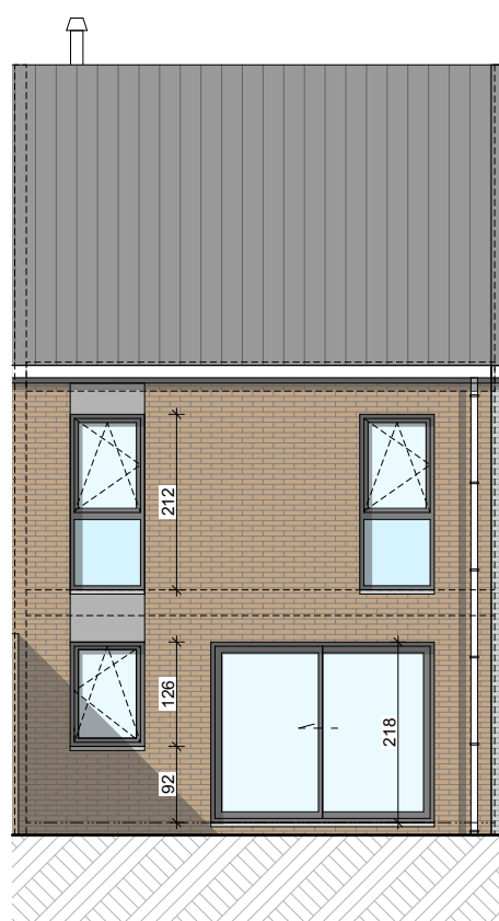
Façade arrière
