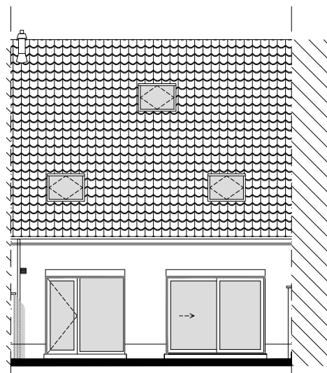
Achtergevel
