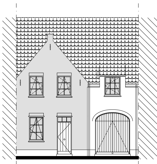
Voorgevel
