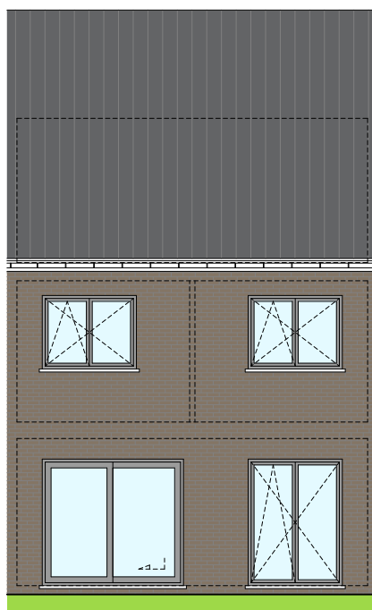
Façade arrière
