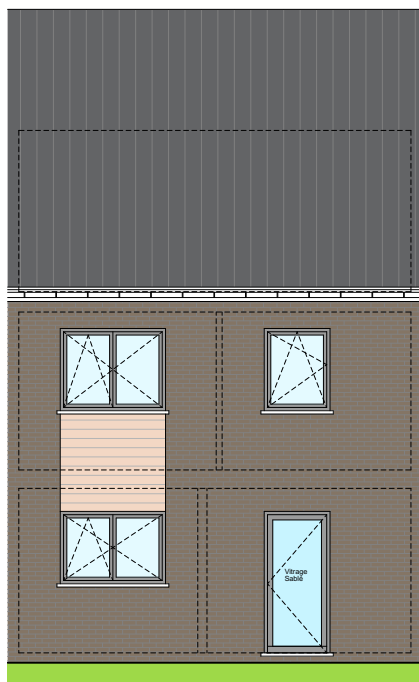
Façade avant
