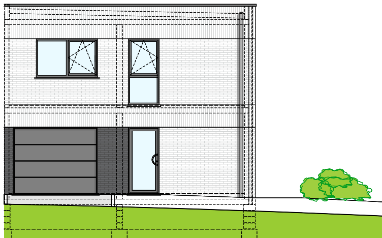
Façade avant
