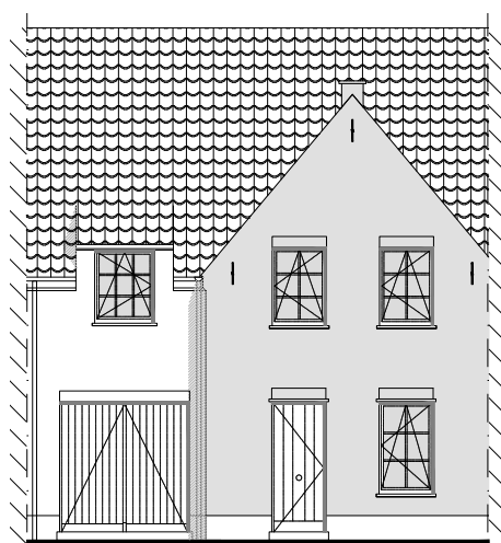
Voorgevel
