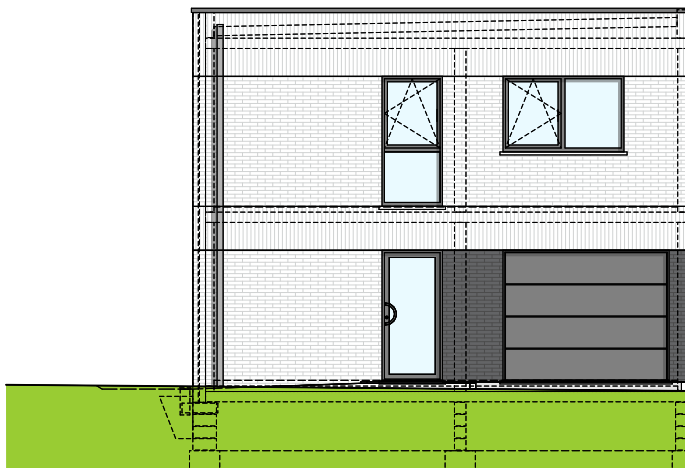
Façade avant
