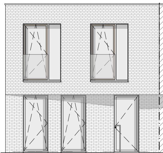
Vorgevel
