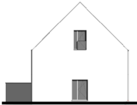
Zijgevel links
