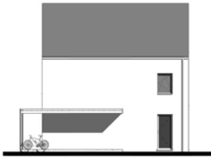
Zijgevel links
