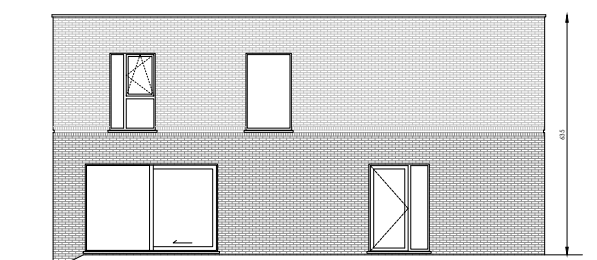
Zijgevel links
