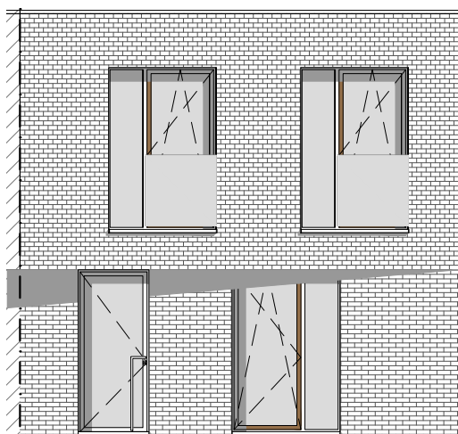
Voorgevel
