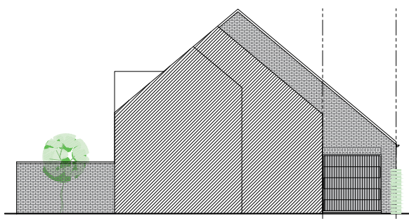
Voorgevel
