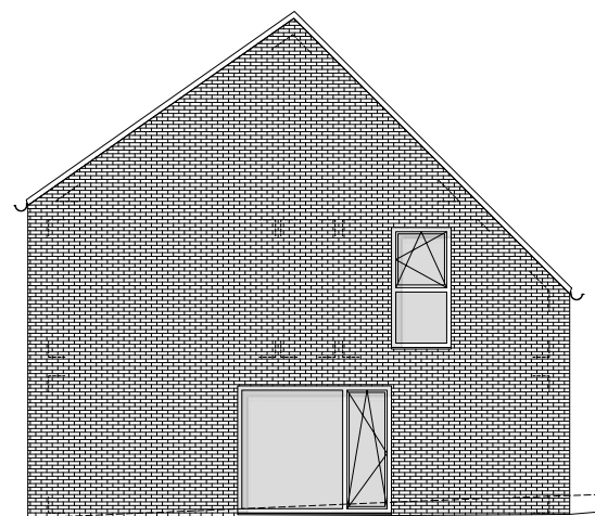
Zijgevel rechts
