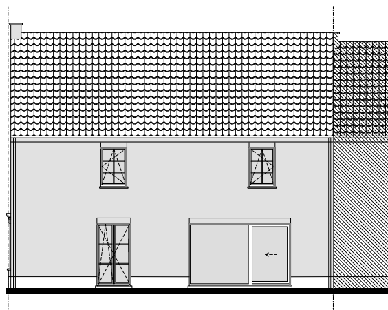
Zijgevel rechts
