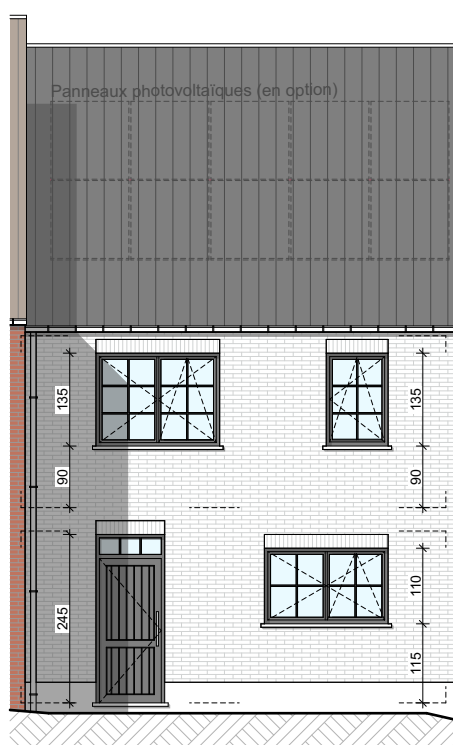
Façade avant
