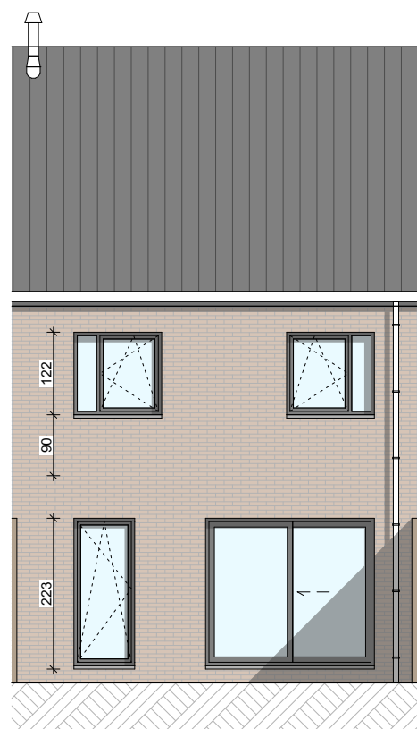
Façade arrière
