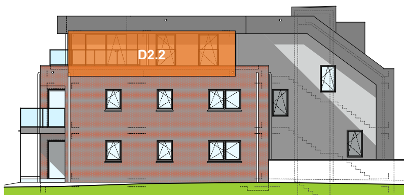
Façade Sud
