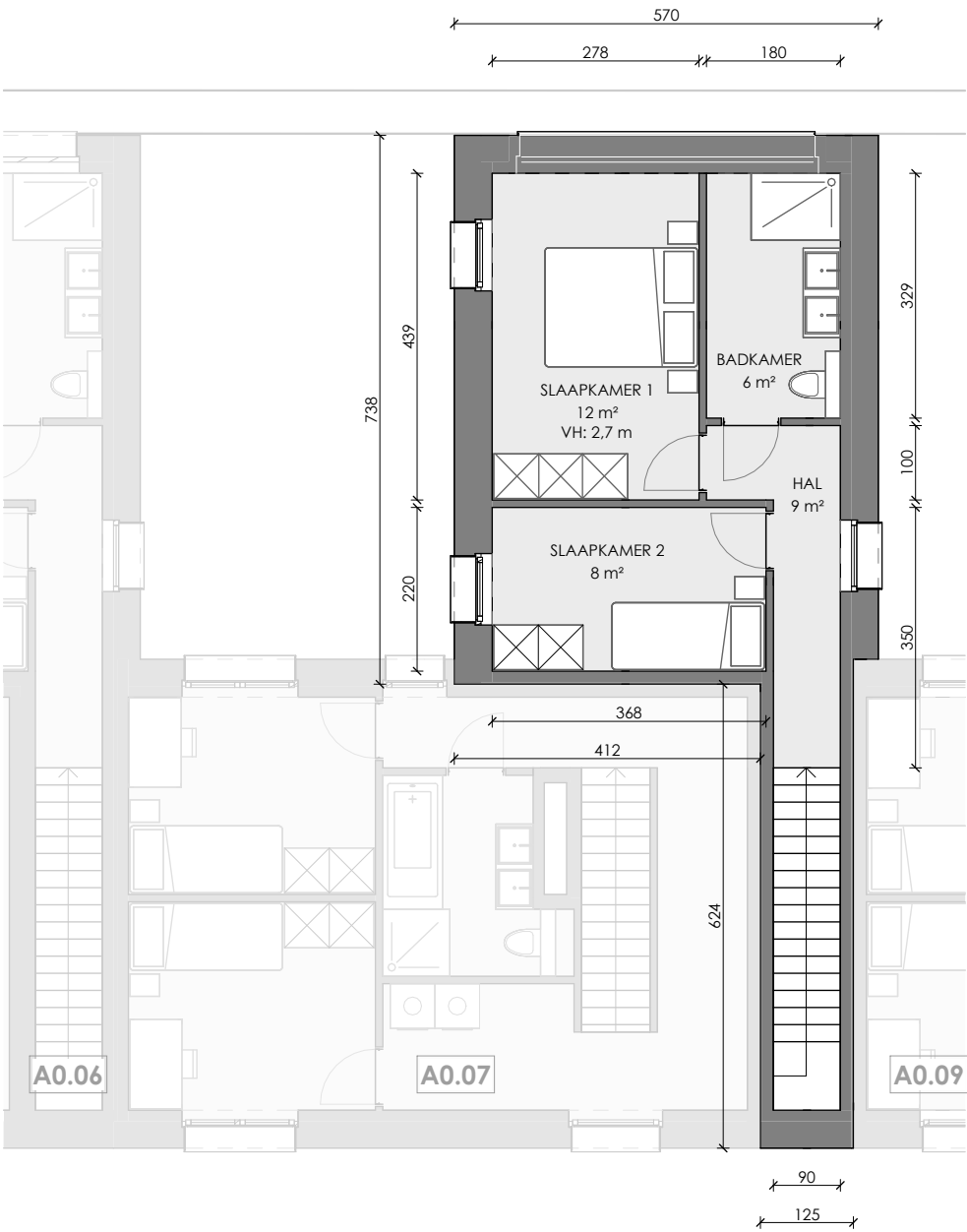
EERSTE VERDIEPING
