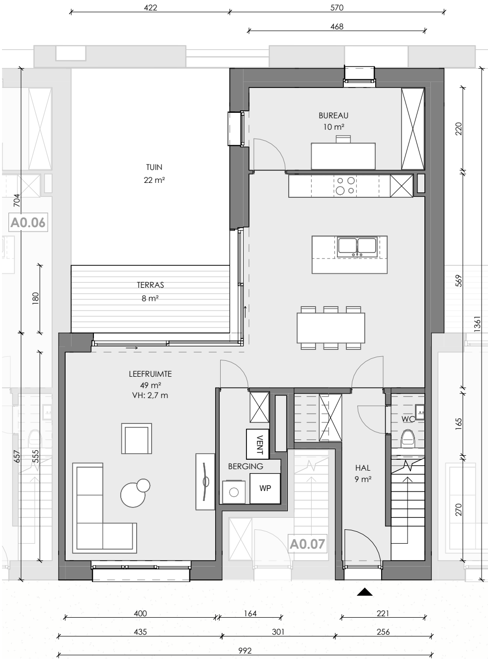
GELUKVLOERS
